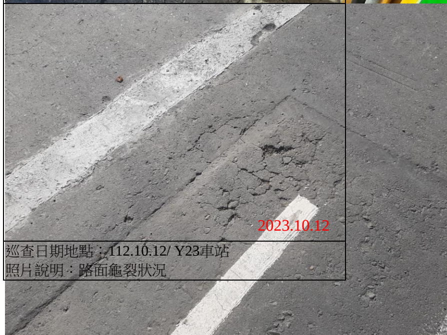
巡查日期地點：112.10.12/ Y23車站 照片說明：路面龜裂狀況
