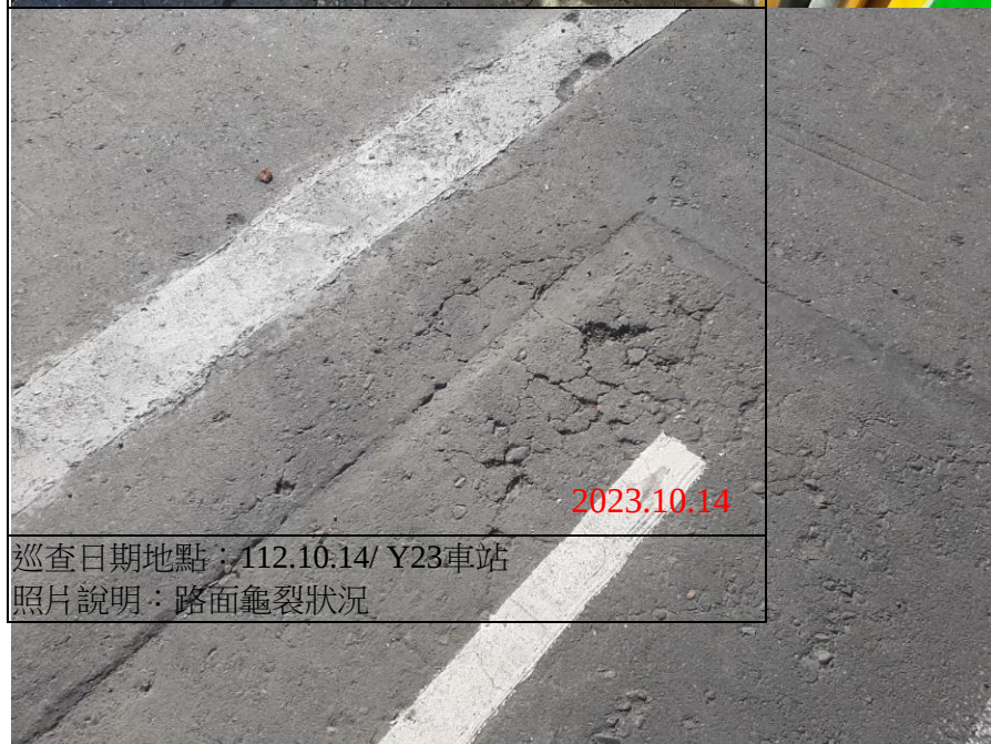
巡查日期地點：112.10.14/ Y23車站 照片說明：路面龜裂狀況
