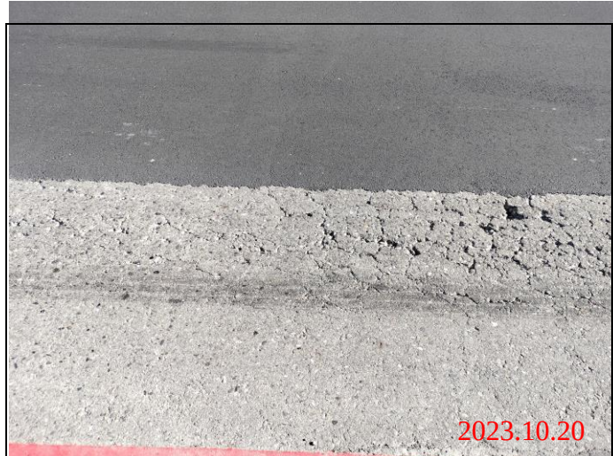
巡查日期地點：112.10.20/ Y23車站 照片說明：路面龜裂狀況
